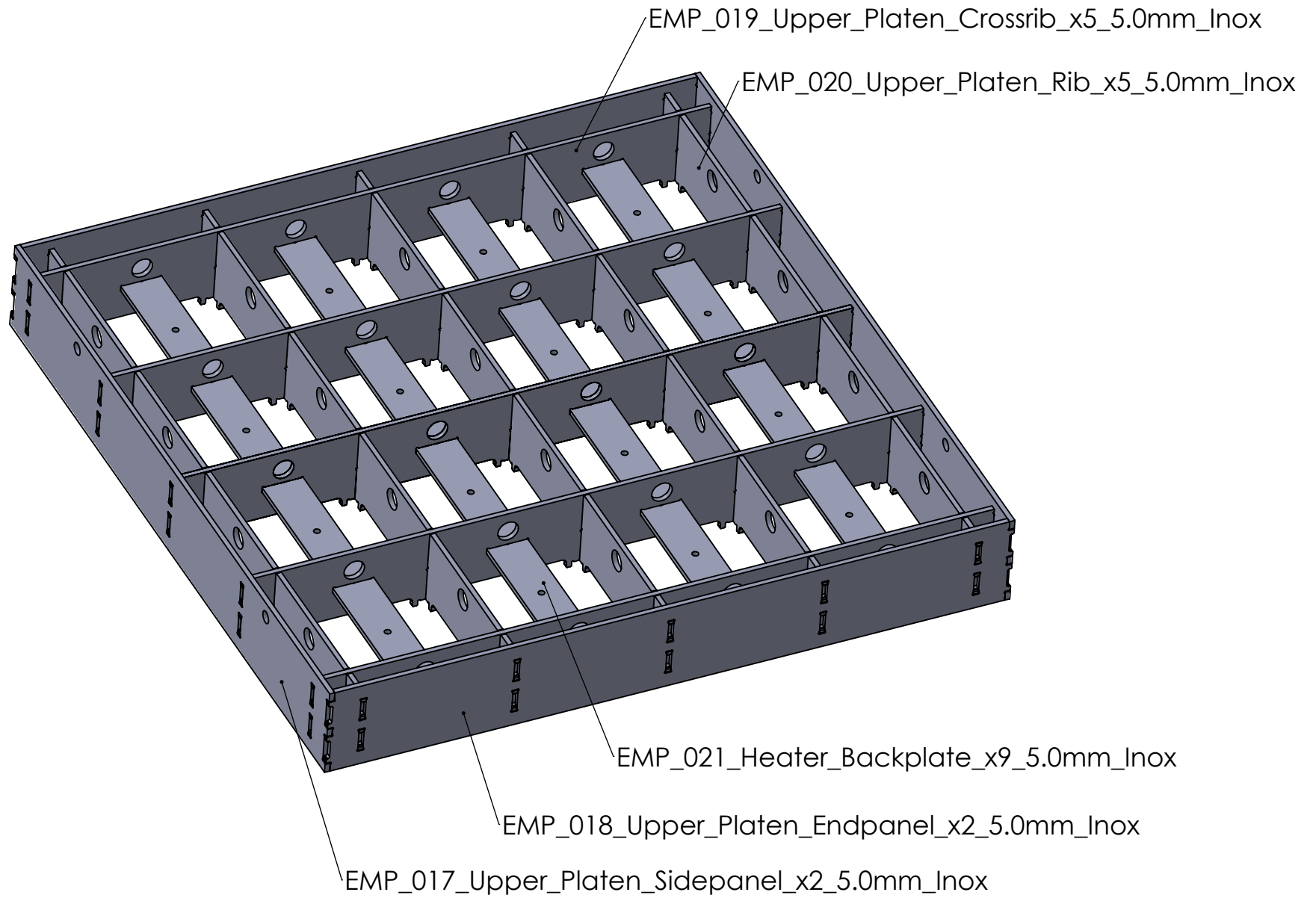
Electric Mini Press - Upper Platten Matrix Assembly
