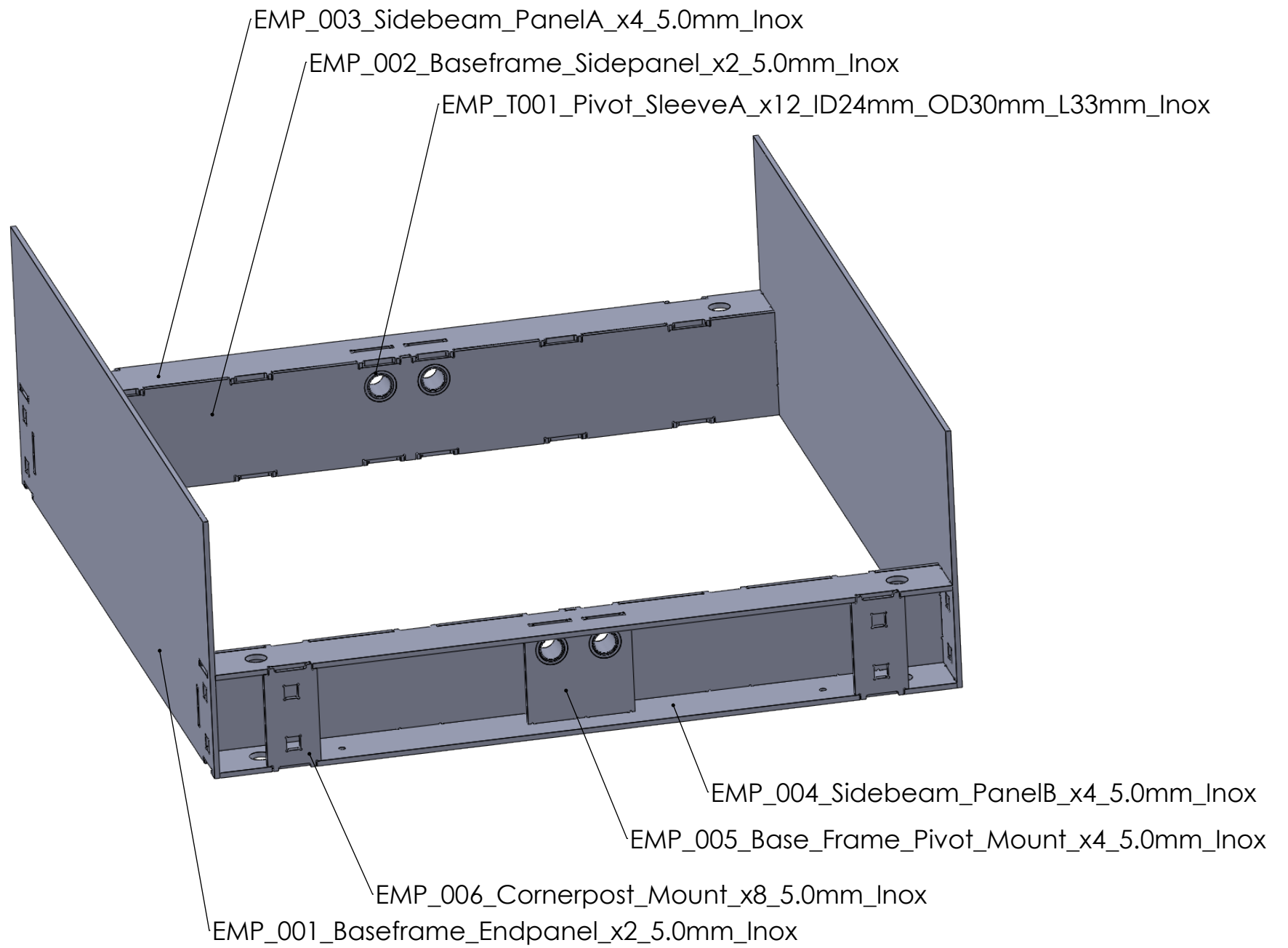
Electric Mini Press - Base Frame Assembly
