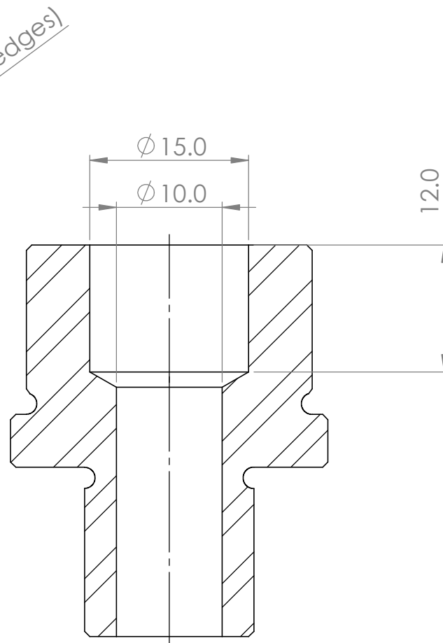
SECTION A-A
