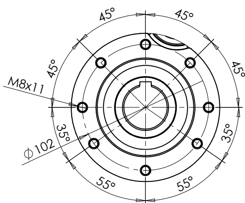
DETALLE B
