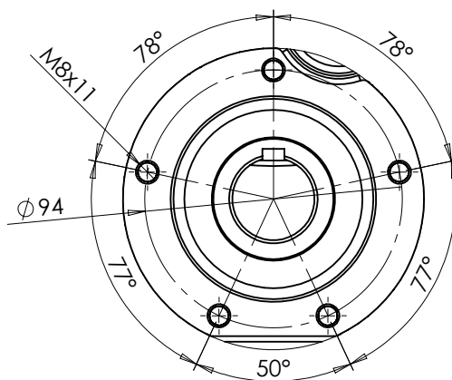
DETALLE B
